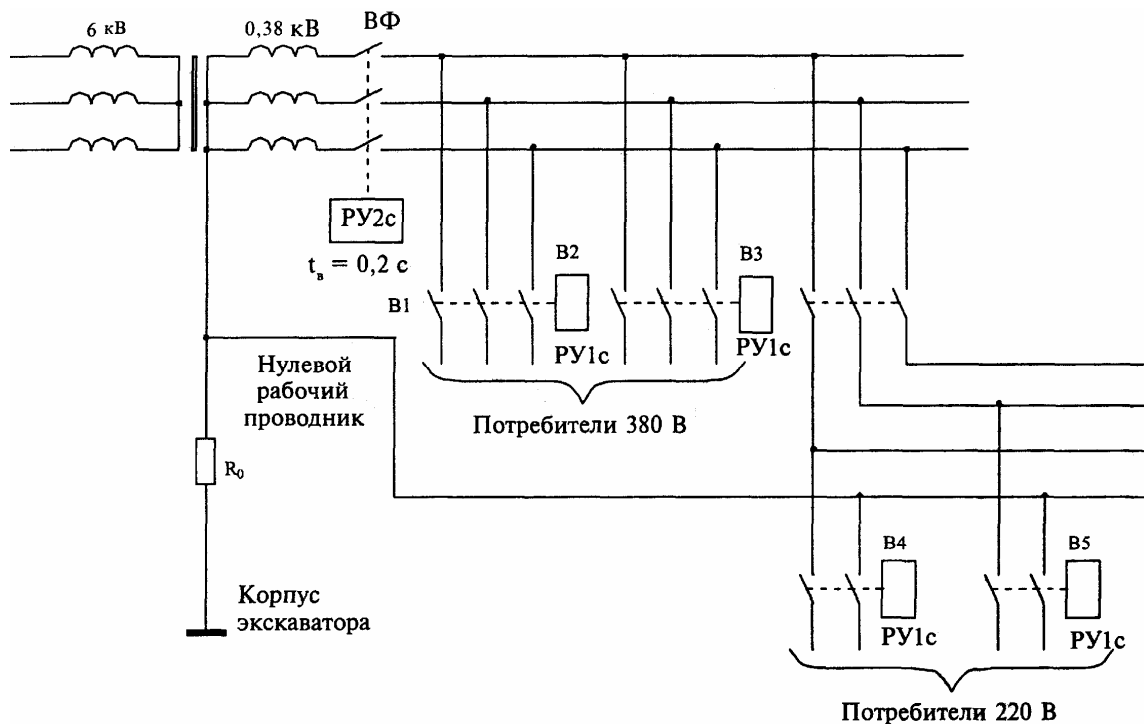
Рис. П.3.1. Схема размещения двухступенчатой защиты
